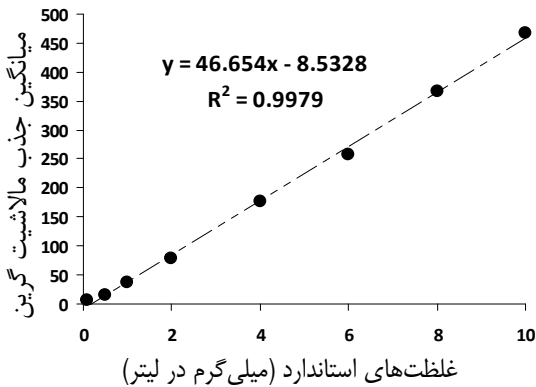
شکل ۱. منحنی استاندارد جذب رنگ مالا شیت گرین در غلظت های استاندارد
