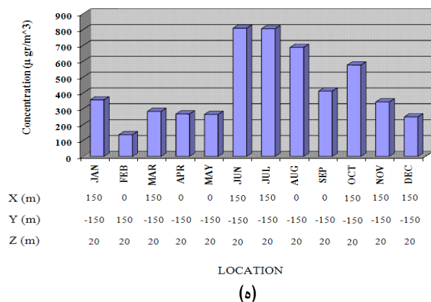
شکل شماره (۵): تغییرات ماهانه بیشترین غلظت ها به همراه زمان و مکان رخداد آنها نسبت به مبدأ انتخابی (الف) متوسط ۱ ساعته (ب) متوسط ۳ ساعته (ج) متوسط ۸ ساعته (د) متوسط ۲۴ ساعته (ه) متوسط یک ماهه
