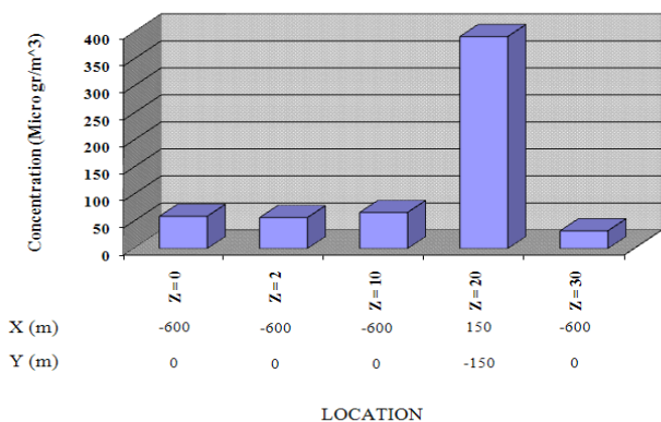
شکل شماره (۶): تغییرات بیشترین غلظت متوسط یک ساله به همراه مکان رخداد آنها نسبت به مبدأ و به تفکیک ارتفاع
