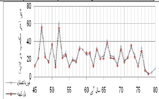
شکل شماره (۲): مقایسه نوسانات دبی سالانه ایستگاه آبسنجی
