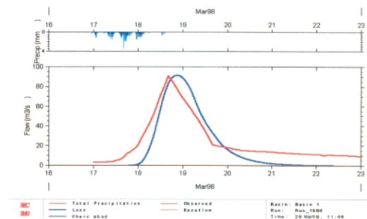
شکل شماره (۳) : هیدروگراف سیلاب محاسبه شده و مشاهداتی رودخانه مرک در محل ایستگاه خرس آباد در اسفند ۱۳۷۶
