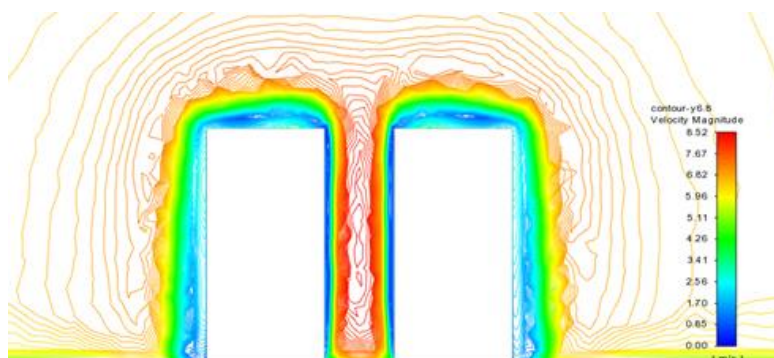
شکل ۸- کانتور سرعت باد در صفحه y=6.8m در کانال ۶ متری
