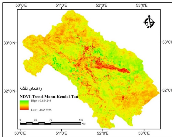
شکل ۴. نقشه روند تغییرات پوشش گیاهی شاخص MODIS-NDVI در حوضه آبخیز گاوخونی طی ۲۰۰۳ تا ۲۰۱۴
