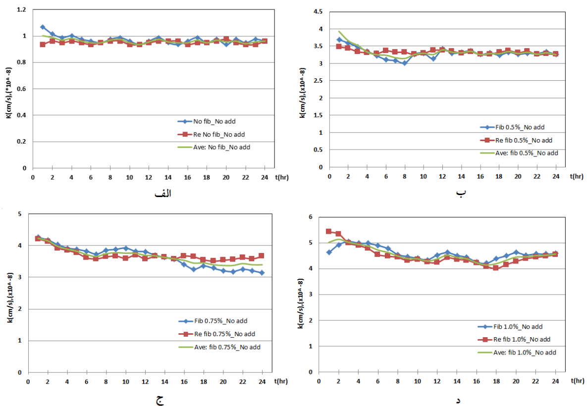
شکل ۴ مقدار ضریب نفوذپذیری به دست آمده با تکرار آزمایش‌ها در نمونه‌هایی با: ۰/۰ درصد الیاف (الف)، ۰/۵ درصد الیاف (ب)، ۰/۷۵ درصد الیاف (ج) و ۱/۰ درصد الیاف (د)
