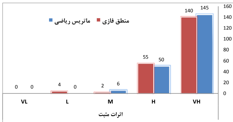
نمودار ۴. مقایسه تعداد اهمیت طبقه‌بندی شده آثار مثبت ارزیابی آثار مرحله اجرای سد کمال صالح در دو روش ماتریس ریاضی و منطق فازی
