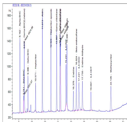
شکل ۲. کروماتوگرام سموم ارگانوکلر در یک نمونه استاندارد
