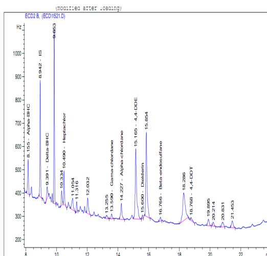
شکل ۳. کروماتوگرام سموم ارگانوکلر در یک نمونه از آب رودخانه
