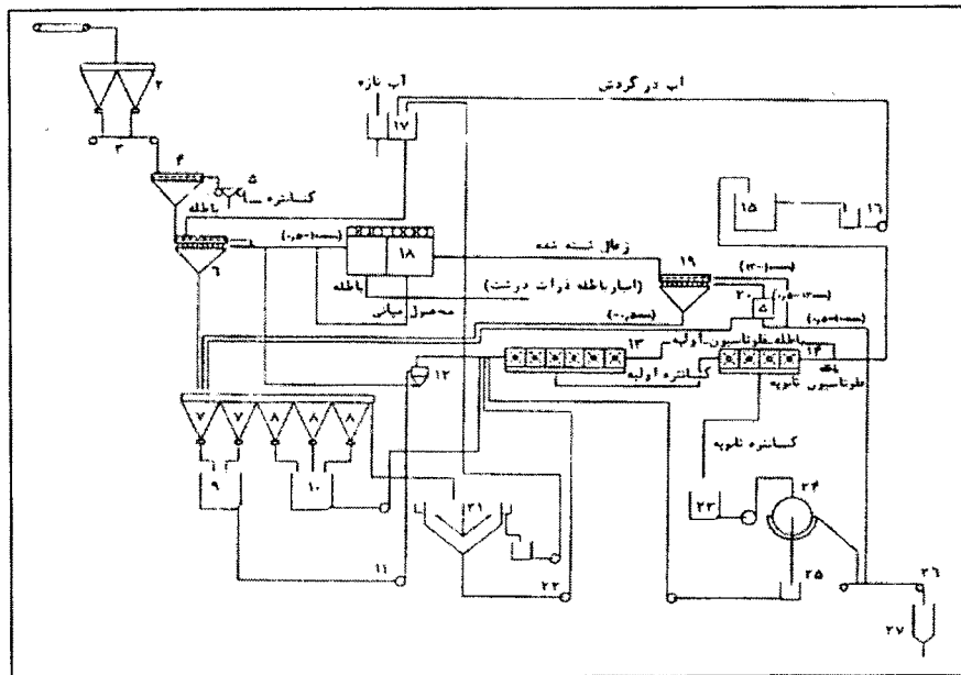
شکل شماره ۲: فلو شیت کارخانه زغالشویی زیر آب
