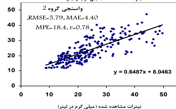
شکل شماره (۵): تغییرات مقادیر نیترات مشاهده شده نسبت به مقادیر پیش بینی شده در آرایش دوم
