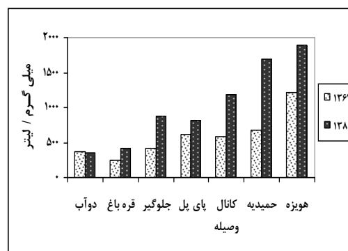
شکل شماره (۶): تغییرات TDS در حوضه آبخیز کرخه
