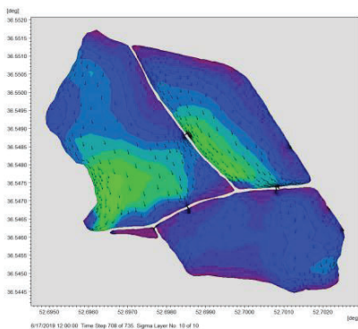
شکل ۴. نتایج مدل در ارتباط با مقایسه جهت و سرعت باد در منطقه و جریان شکل گرفته در سطح آب تالاب
