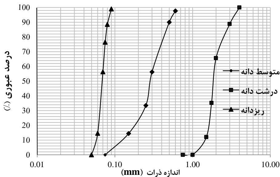
شکل ۲. منحنی دانه‌بندی نمونه‌های رسوبات
