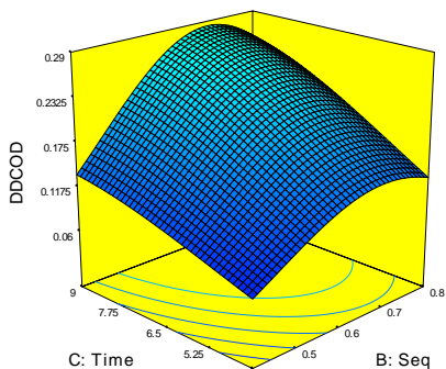
شکل ۵. رابطه بین زمان کلی اعمال امواج فراصوت و تابش غیرپیوسته با درجه تخریب در توان و غلظت لجن ثابت
