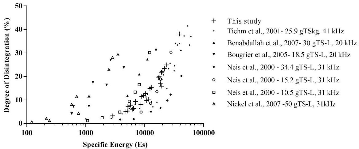
شکل ۱۰. مقایسه بین رابطه انرژی مخصوص و درجه تخریب در تحقیق حاضر و مقاله‌های قبلی
