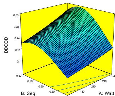
شکل ۲. تأثیر متقابل توان اعمالی و تابش منقطع روی درجه تخریب در زمان و غلظت لجن ثابت
