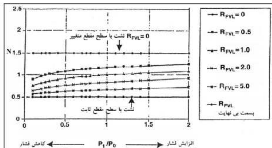
شکل ۱. رابطه بين نسبت فشار و مقدار N در نظریه FAVAD (نشریه ۵۵۶، ۱۳۹۱)
