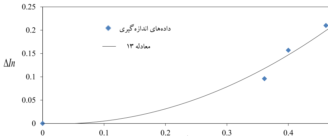
شكل ۶. تغييرات نسبى کاهش ديبى ورودى به ايزوله و فشار خروجى شير فشارشكن
