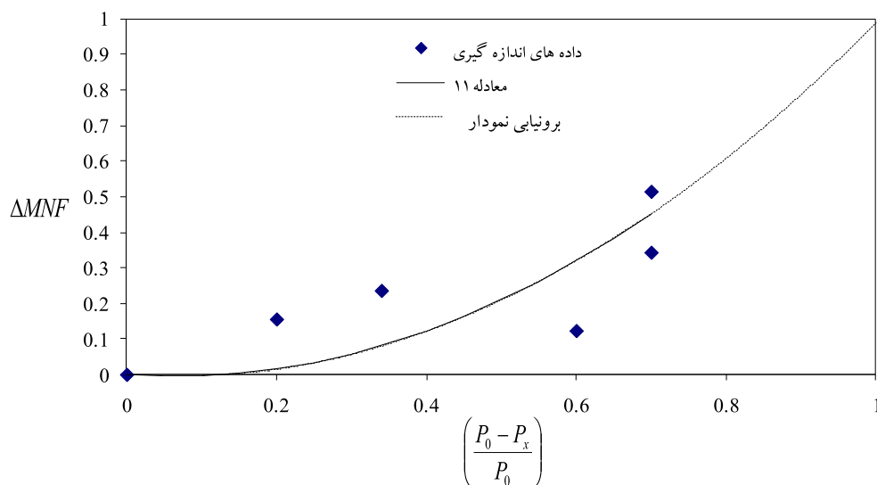
شکل ۴. تغييرات نسبی حداقل جريان شبانه در برابر فشار خروجی شیر فشارشکن
