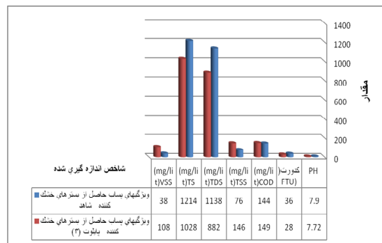
نمودار شماره (۸): مقایسه ویژگی‌های بساب دو بستر ضمن کاهش ضخامت لایه به ۱/۳ ضخامت بستر شاهد و استفاده از لایه‌ای از گونی کنفی
