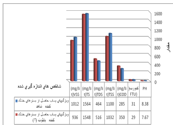
نمودار شماره (۲): مقایسه ویژگی‌های پساب بسترهای شاهد و بستر با مکش هیدرواستاتیکی
