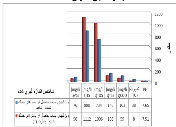
نمودار شماره (۴): مقایسه ویژگی‌های پساب حاصل از بسترهای خشک کننده شاهد و لجن آمایش شده
