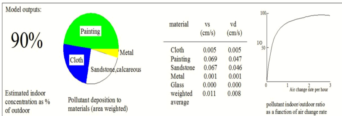
شکل شماره (۹): نتایج مدل IMPACT برای غلظت O 3 در موزه فرش ایران
