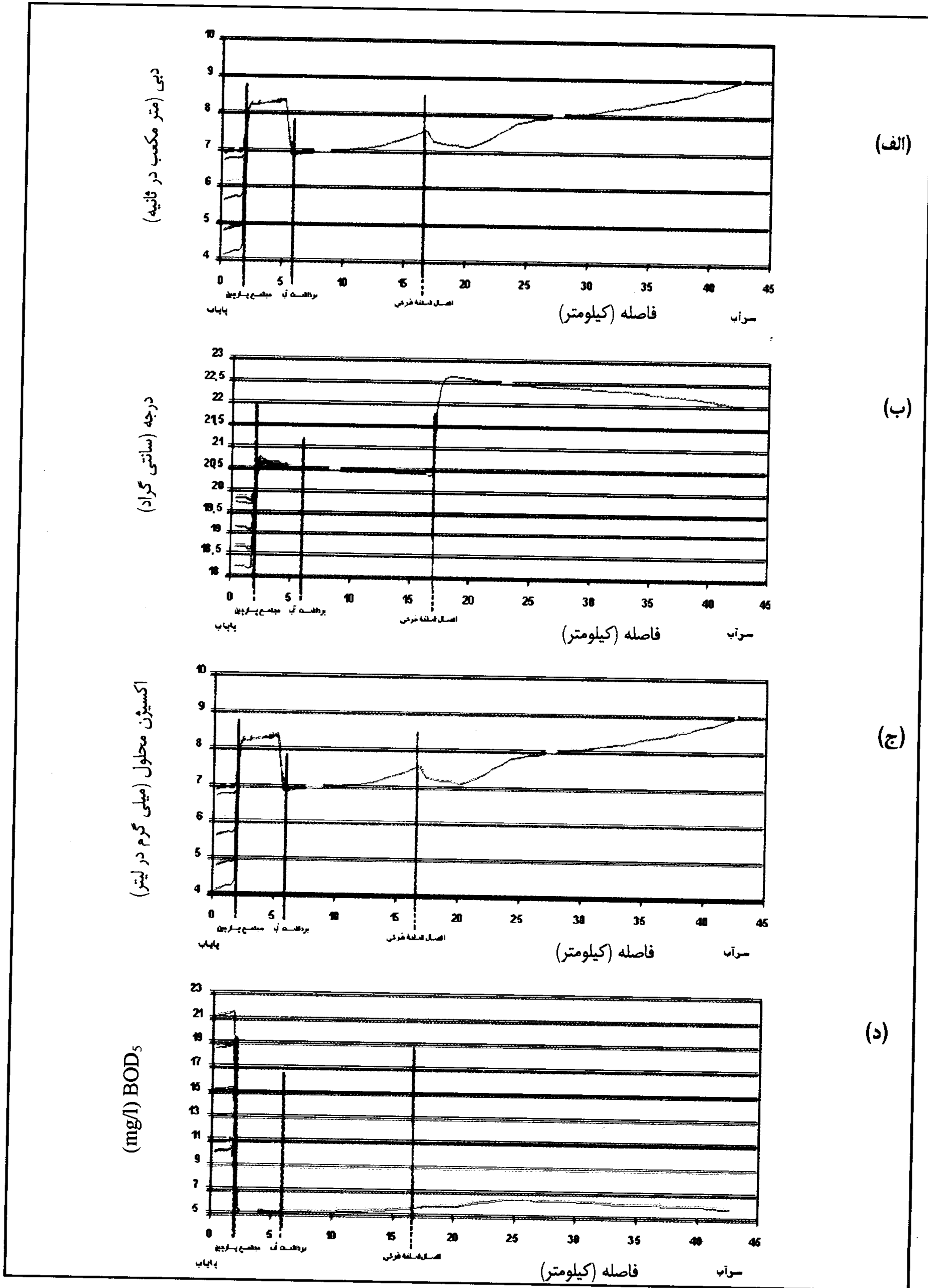
شکل (۲) تغییرات (الف) دیسی، (ب) درجه حرارت، (ج) غلظت اکسیژن محلول و (د) اکسیژن خواهی پنج روزه در طول شاخه اصلی رودخانه در تیرماه به ازای ۱، ۲، ۳، ۴، ۵ و ۵ متر مکعب در ثانیه برداشت آب.
