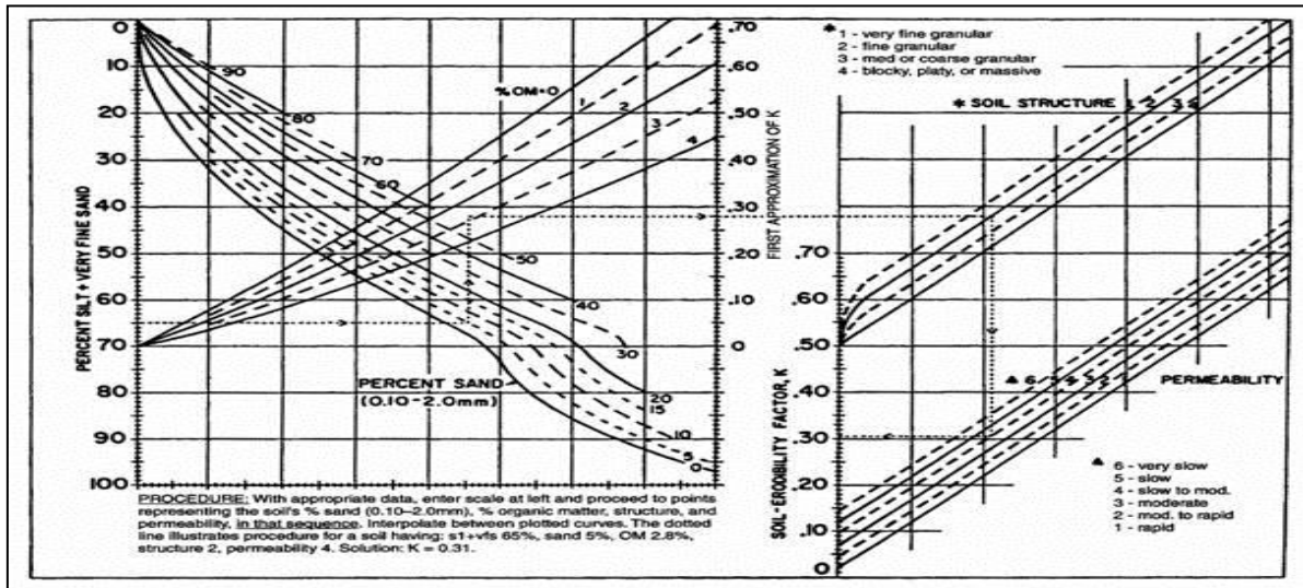
شکل ۲. نمودار برآورد میزان فرسایش پذیری خاک در مدل RUSLE
