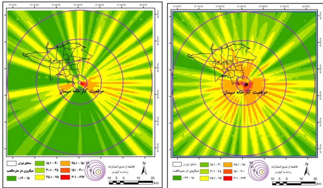
شکل ۵. آلودگی پراکنش و غلظت آلاینده ذرات معلق برای متوسط یک ساعته تابستانه (راست) زمستانه (چپ)
