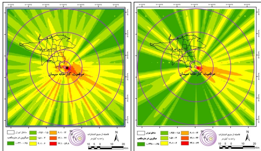
شکل ۶. آلودگی پراکنش و غلظت آلاینده ذرات معلق (PM 10 ) برای متوسط روزانه تابستانه (راست) زمستانه (چپ)
