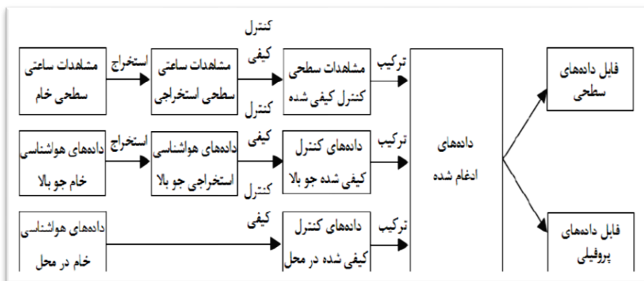
شکل ۳. فرایند آماده‌سازی اطلاعات برای AERMOD با پیش‌پردازنده AERMET منبع: EPA, 2004
