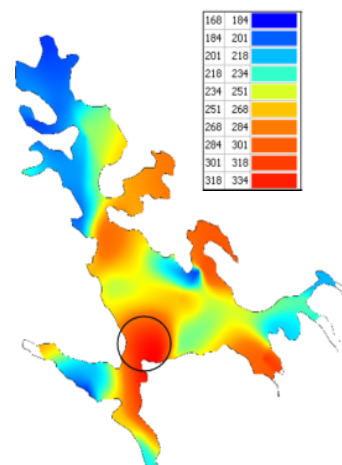
شکل شماره (۴): پهنه بندی سختی آب دشت
