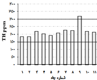
نمودار شماره (۶): سختی کل در بهار ۸۳
