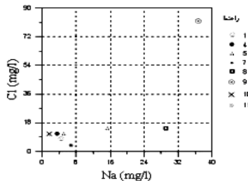
شکل شماره (۸): دیاگرام برابری غلظت‌های سدیم و کلر
