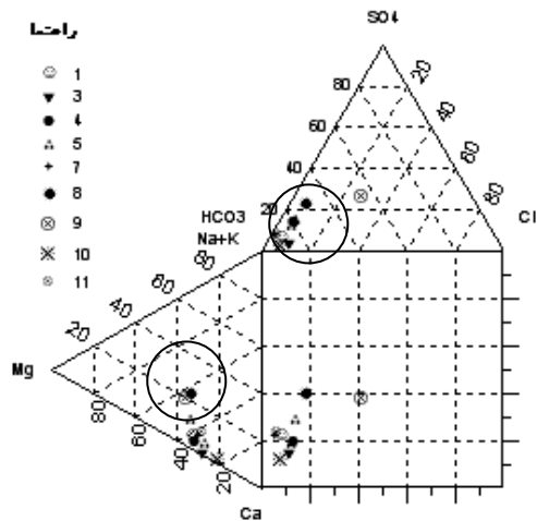
شکل شماره (۷): نسبت یون‌ها در تشکیلات شیمیایی آب
